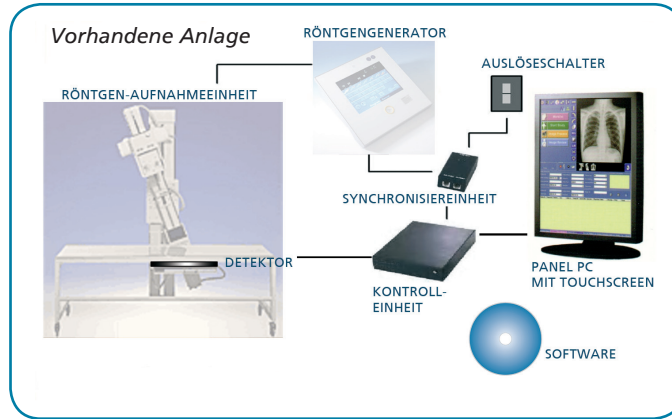
STARMEDPRO DR set bestehend aus: Panel PC, Kontroll- und Synchronisiereinheit, Auslöseschalter, Detektorgehäuse mit verschiedenen Detektoren zur Auswahl.
